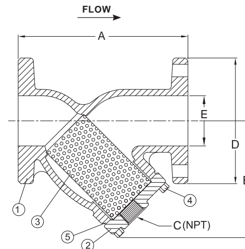
F-721-A Flanged
